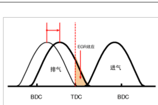
(4) 高速/高负荷
