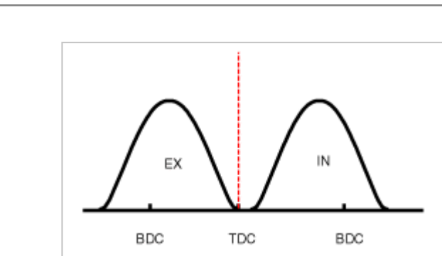
(3) 低速/高负荷
